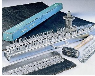
Uniones para bandas ligeras, por medio de un útil de colocación a martillo
